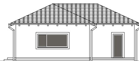
POHLED P4
